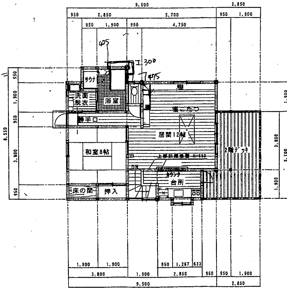
二階平面図
