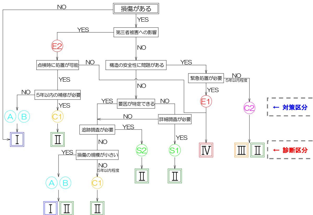
▲図 2-8-1. 診断区分選定フロー（案）
