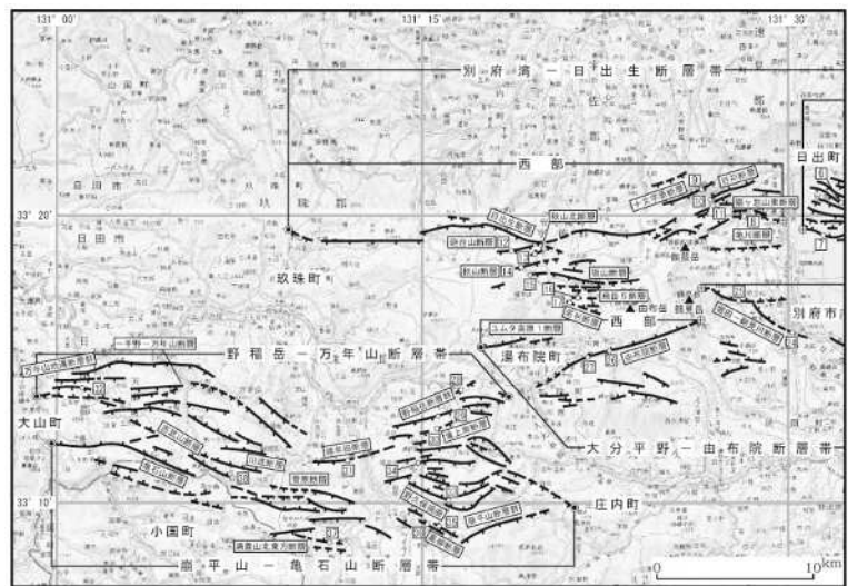
図 「野稻岳一万年山断層帯」「崩平山-亀石山断層帯」
