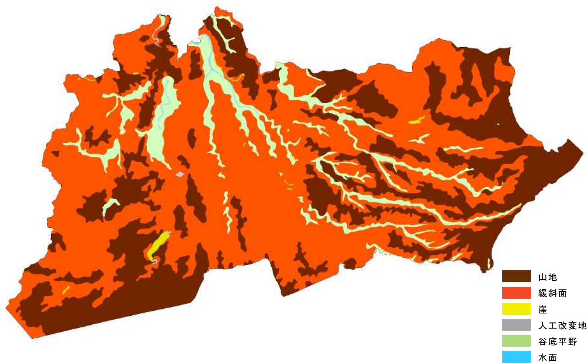
図 南小国町の地形
