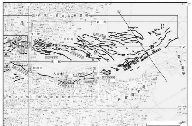
図 「別府湾一日出生断層帯」「大分平野一由布院断層帯」
