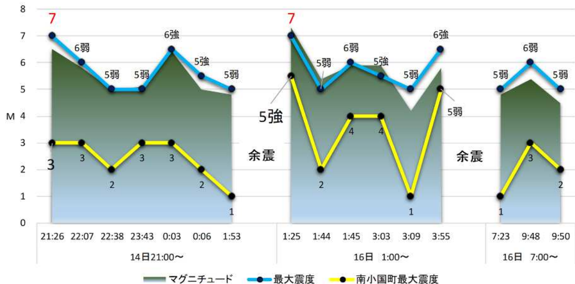
図 4月14日～16日午前までに発生した地震(震度5以上)と南小国町の震度推移図
