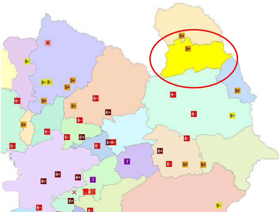
図 熊本地震(4月16日1:25発生 マグニチュード7.3)における南小国町の震度
