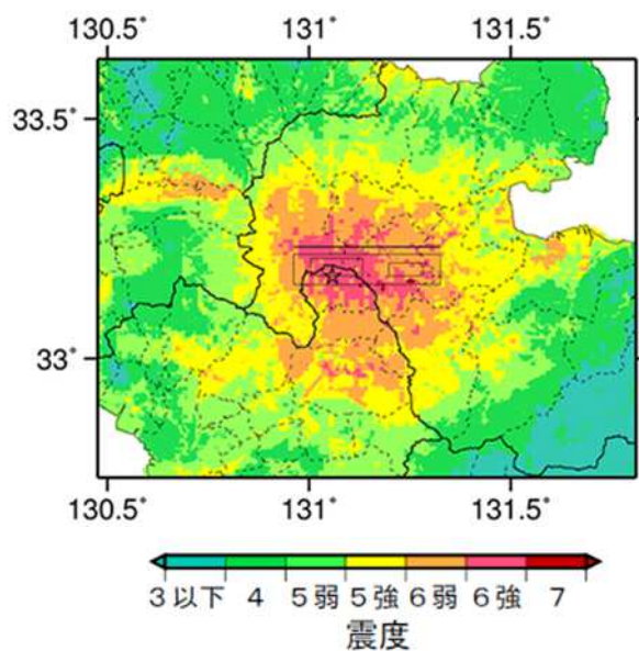
図 野稲岳一万年山断層帯震源の震度分布図
