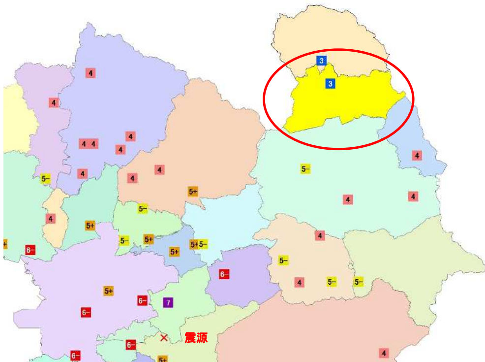
図 熊本地震(4月14日21:26発生 マグニチュード6.5)における南小国町の震度
